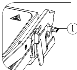
① --- Levier de déblocage des charnières
